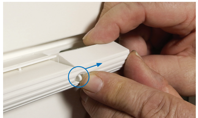
Pikakiinnitteisen venttiiliyksikön vapautinvipu
